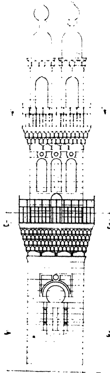
واجهة المئذنة
